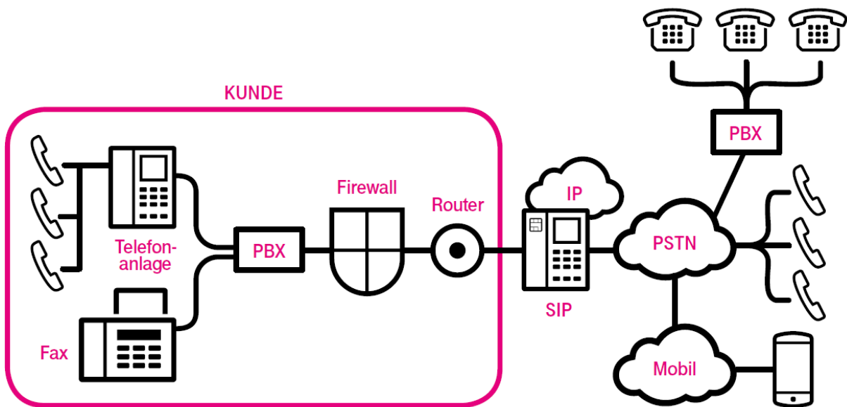
Abbildung 1 - Prinzipdarstellung einer Anbindung über SIP Trunk
