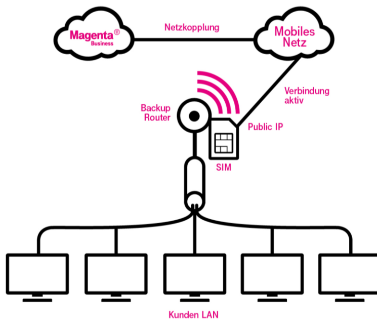
Abbildung 1: Quick Install
